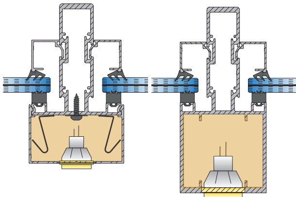
LED-Beleuchtung mittels Aufklipp-Profil
